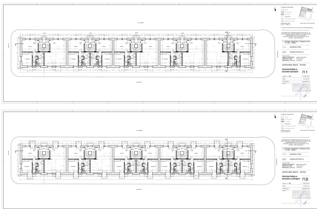
Σχέδιο 3) Πολυκατοικία Α: Κάτοψη Ισογείου και Α Ορόφου (αντίγραφο από εγκεκριμένα σχέδια μελέτης)
