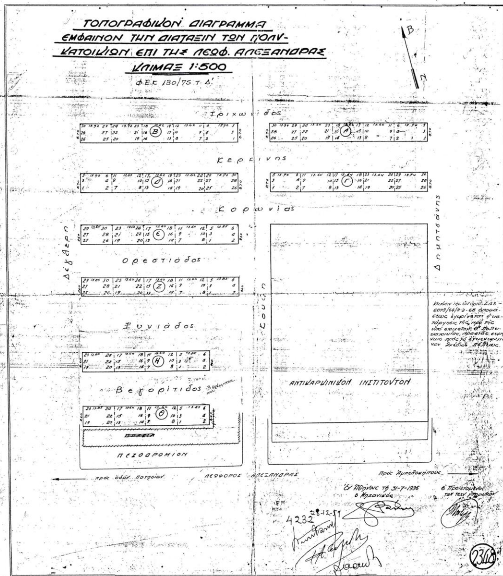
Σχέδιο 4) Τοπογραφικό Διάγραμμα 1936
