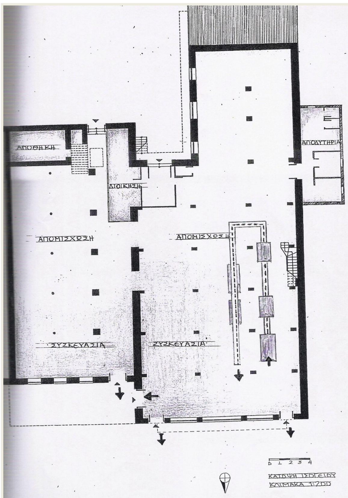
ΙΣΟΓΕΙΟ: ΑΠΟΜΙΣΧΩΣΗ ΚΑΙ ΣΥΣΚΕΥΑΣΙΑ ΠΡΟΙΟΝΤΟΣ-ΕΞΟΔΟΣ ΑΠΟ ΤΗΝ ΠΛΕΥΡΑ ΤΗΣ ΠΡΟΚΥΜΑΙΑΣ
