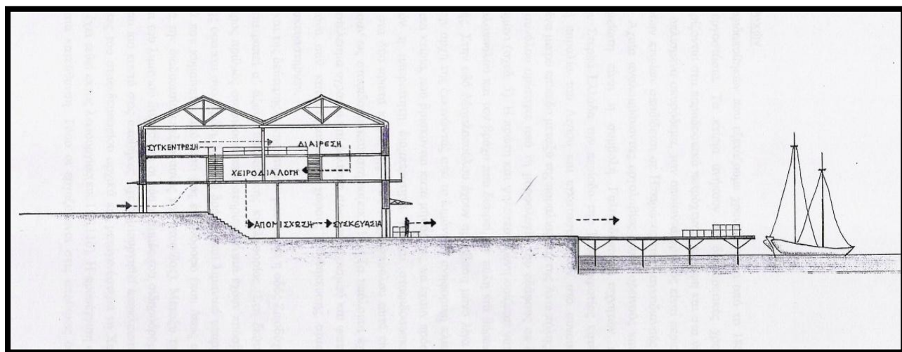
ΔΙΑΔΡΟΜΗ ΣΤΑΦΙΔΟΚΑΡΠΟΥ ΣΕ ΤΡΙΩΡΟΦΟ ΣΤΑΦΙΔΕΡΓΟΣΤΑΣΙΟ
