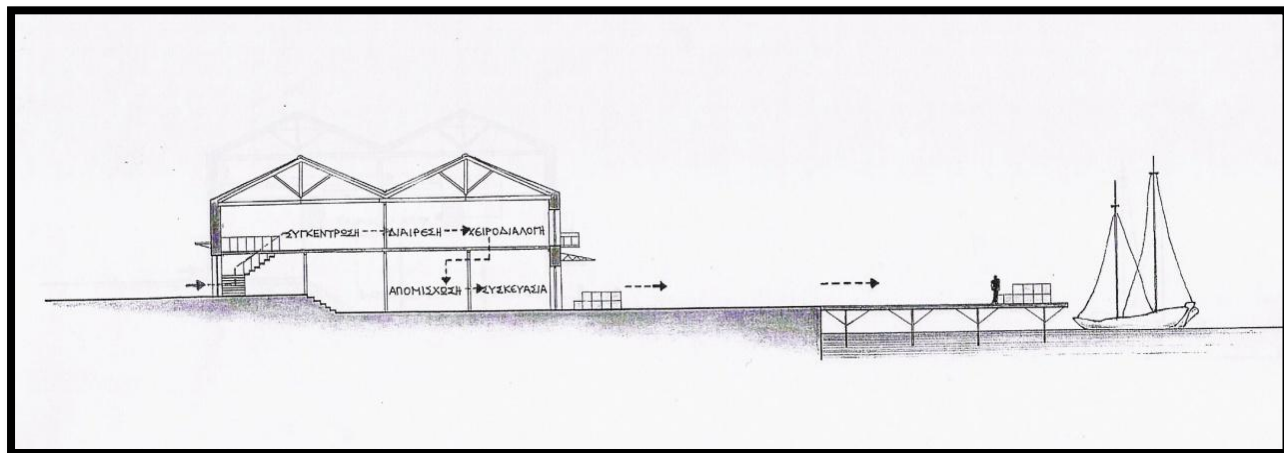
ΔΙΑΔΡΟΜΗ ΣΤΑΦΙΔΟΚΑΡΠΟΥ ΣΕ ΔΙΩΡΟΦΟ ΣΤΑΦΙΔΕΡΓΟΣΤΑΣΙΟ
