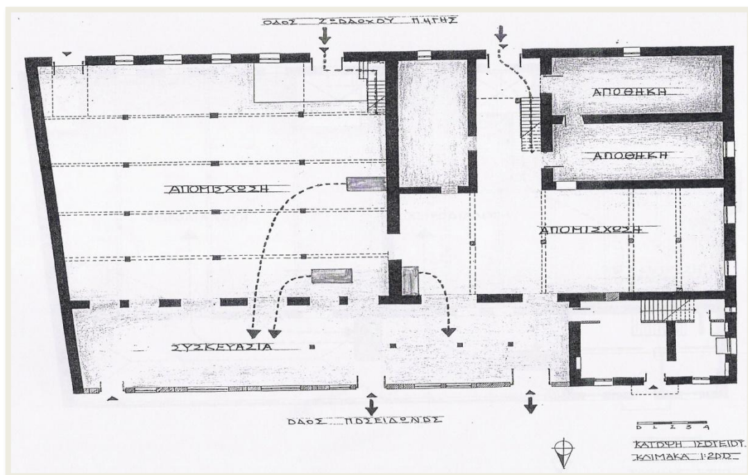
ΙΣΟΓΕΙΟ: ΑΠΟΜΙΣΧΩΣΗ ΚΑΙ ΣΥΣΚΕΥΑΣΙΑ-ΕΞΟΔΟΣ ΑΠΟ ΤΗΝ ΟΔΟ ΠΟΣΕΙΔΩΝΟΣ
