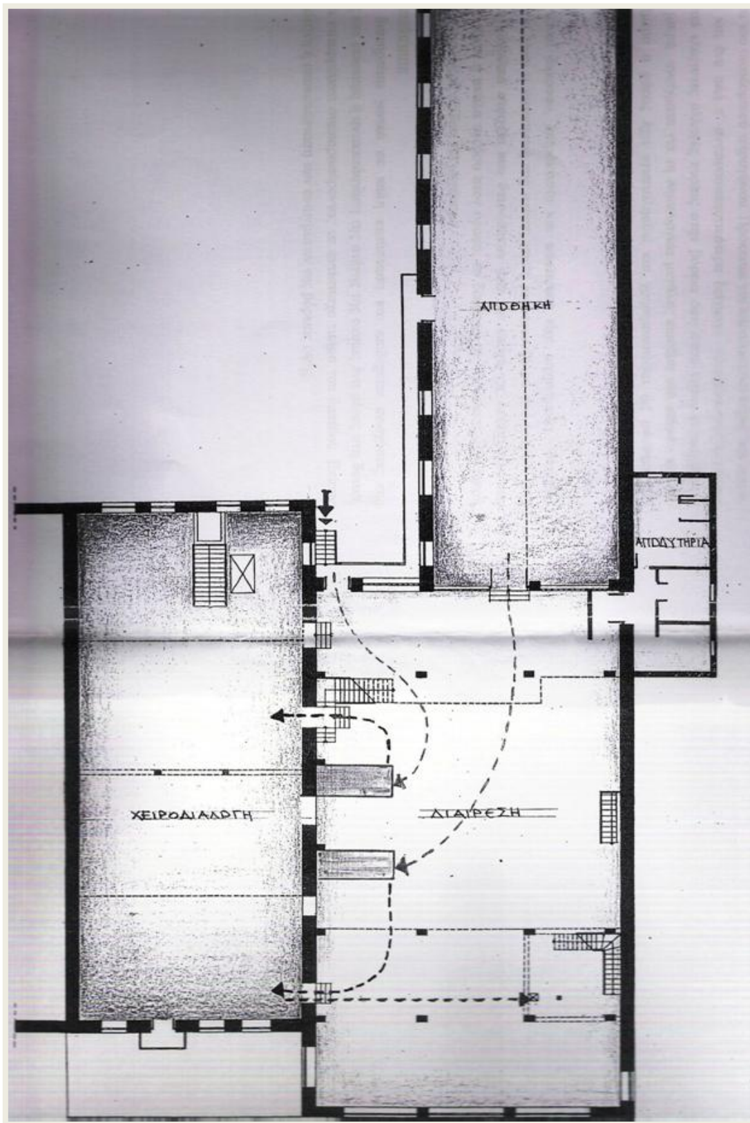
ΕΙΣΟΔΟΣ ΣΤΑΦΙΔΑΣ ΑΠΟ ΤΗΝ ΟΔΟ ΠΑΥΣΑΝΙΟΥ ΣΤΗΝ ΑΠΟΘΗΚΗ ΤΟΥ ΠΡΩΤΟΥ ΟΡΟΦΟΥ: ΔΙΑΙΡΕΣΗ ΚΑΙ ΧΕΙΡΟΔΙΑΛΟΓΗ
