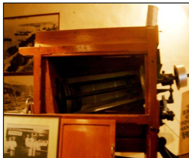
«ΚΛΙΝΑΡΙΣΤΙΚΗ» -ΑΠΟΜΙΣΧΩΤΙΚΗ ΜΗΧΑΝΗ
