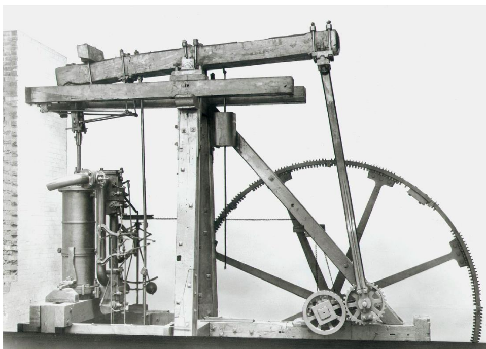
Εικόνα 2. Ατμομηχανή σχεδιασμένη και κατασκευασμένη από τους James Watt (1736-1819) και Matthew Boulton (1728-1809). Μια από τις βασικές καινοτομίες της Βιομηχανικής Επανάστασης. Χρονολογείται από το 1788. Η παλαιότερη αρχική περιστροφική ατμομηχανή στον κόσμο. Science Museum, London.
