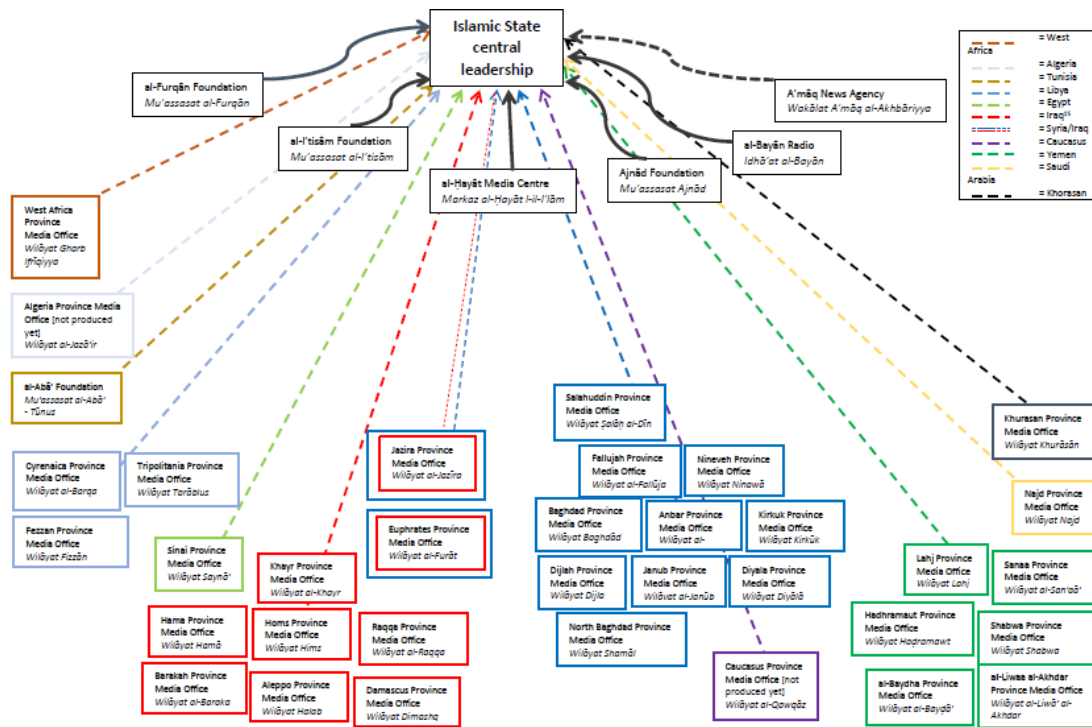
Εικόνα 6.1: Τα δίκτυα προπαγάνδας του ISIS ανά τον κόσμο
