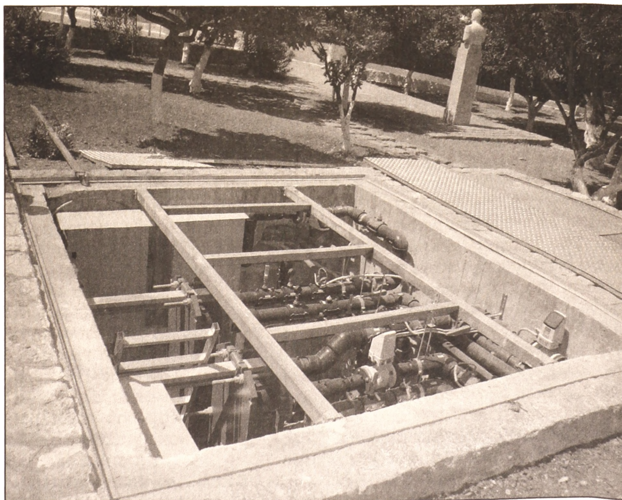
Κεντρικό δημοτικό ψυγείο (Υδρα 2003).
