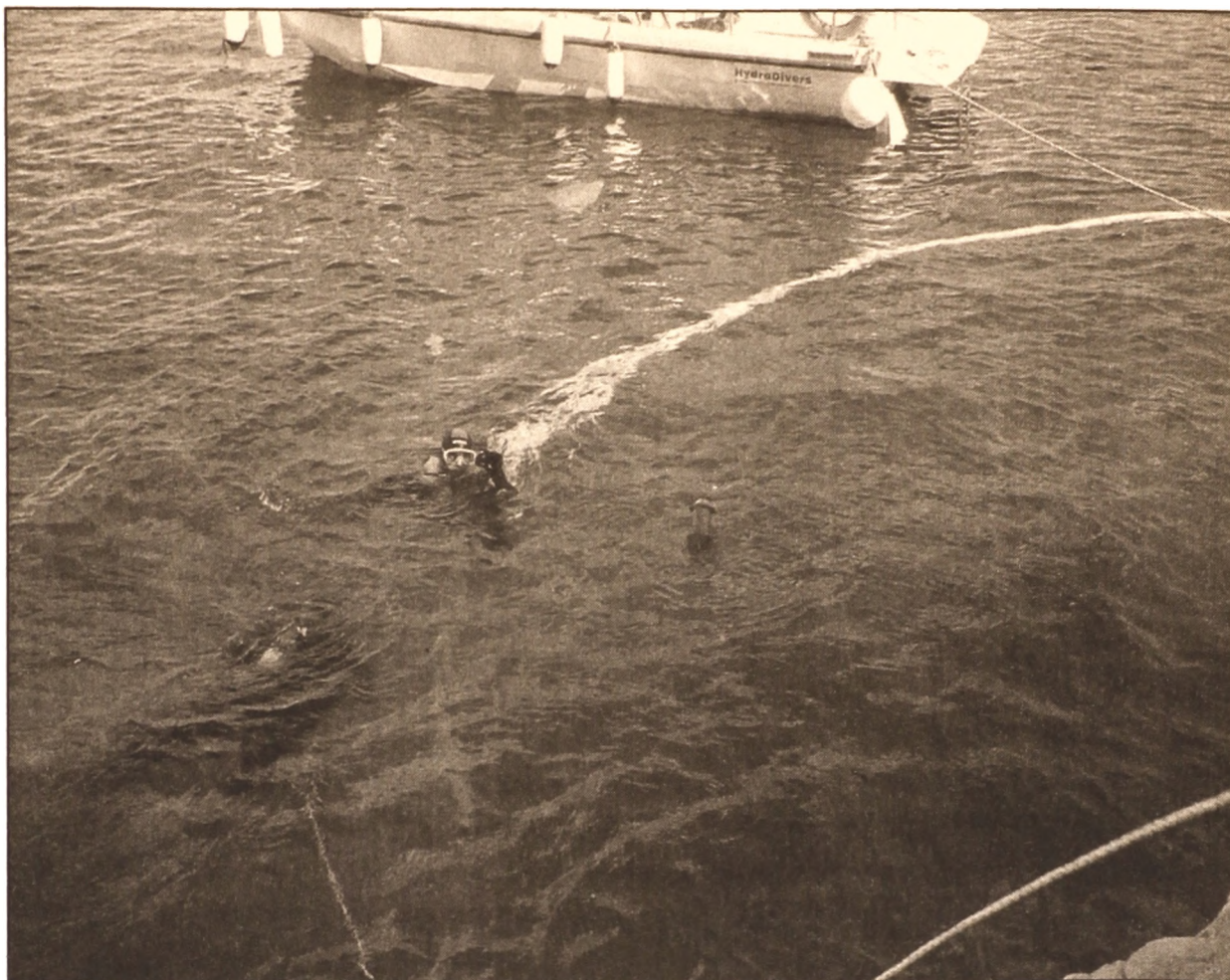
Σύνδεση υποθαλάσσιου αγωγού για την άντληση θαλασσινού νερού προς κλιματιστικές μονάδες (Υδρα 2003).
