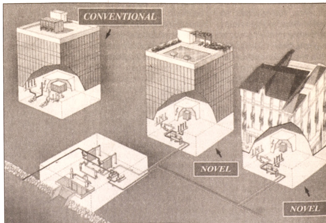
Σύγκριση συμβατικού κεντρικού συστήματος κλιματισμού (αερόψυκτα μηχανήματα) με υδρόψυκτα από θάλασσα μηχανήματα.
