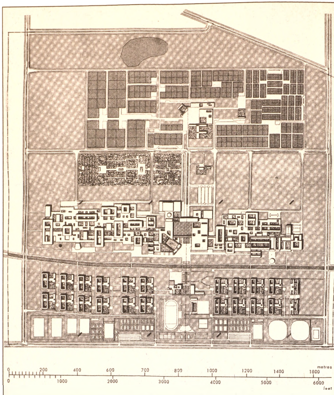
Εικ. 6. Πανεπιστήμιο του Punjab, σχέδιο γενικής διάταξης.
