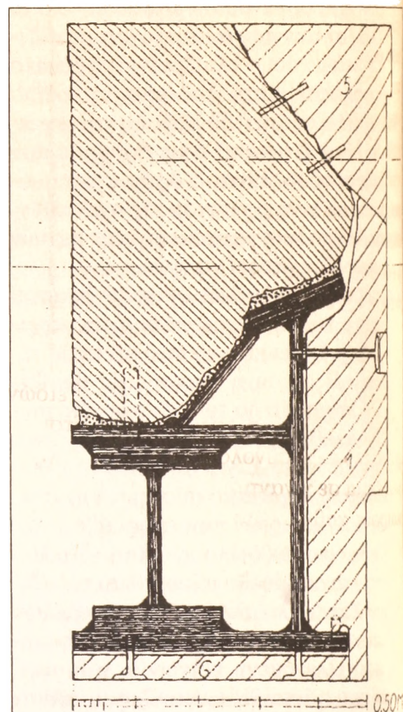
Πρόταση αποκατάστασης υπέρθυρου διακοσμικής θύρας Παρθενώνα (Μ. Κορρές)
