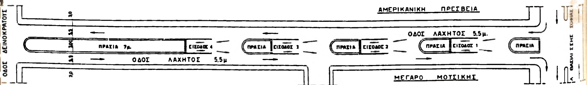
ΟΡΙΖΟΝΤΙΟΓΡΑΦΙΑ ΟΔΟΥ ΛΑΧΗΣ (1:500)
