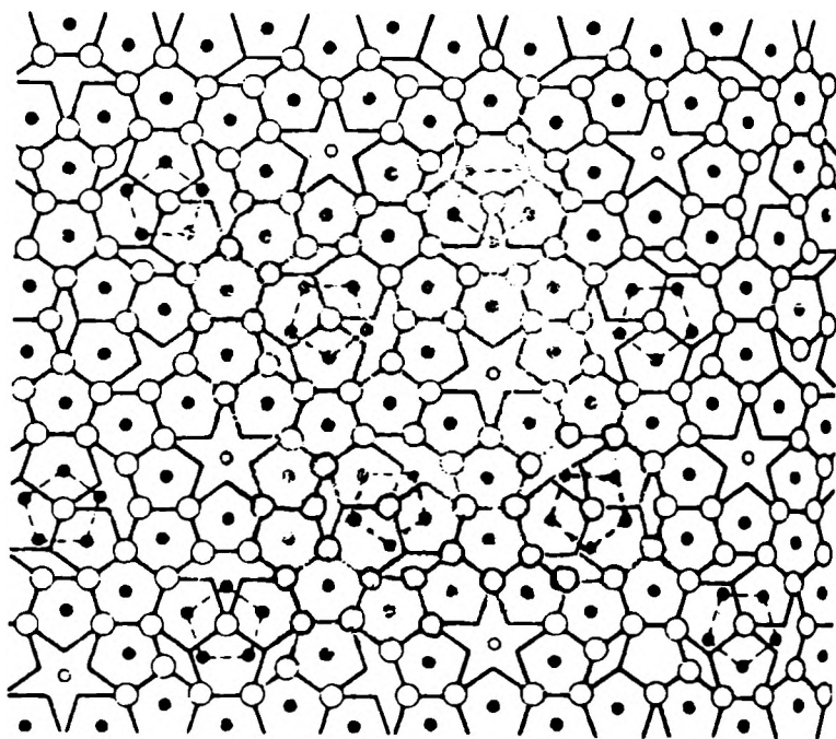
Δομή των ημικρυστάλλων όπως προτείνεται από τους ερευνητές των Bell Labs της AT&T. Η πενταπλή συμμετρία είναι εμφανής.
