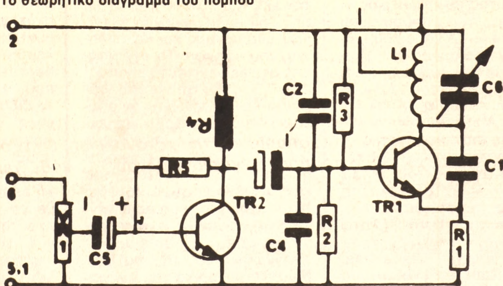
Το θεωρητικό διάγραμμα του πομπού
