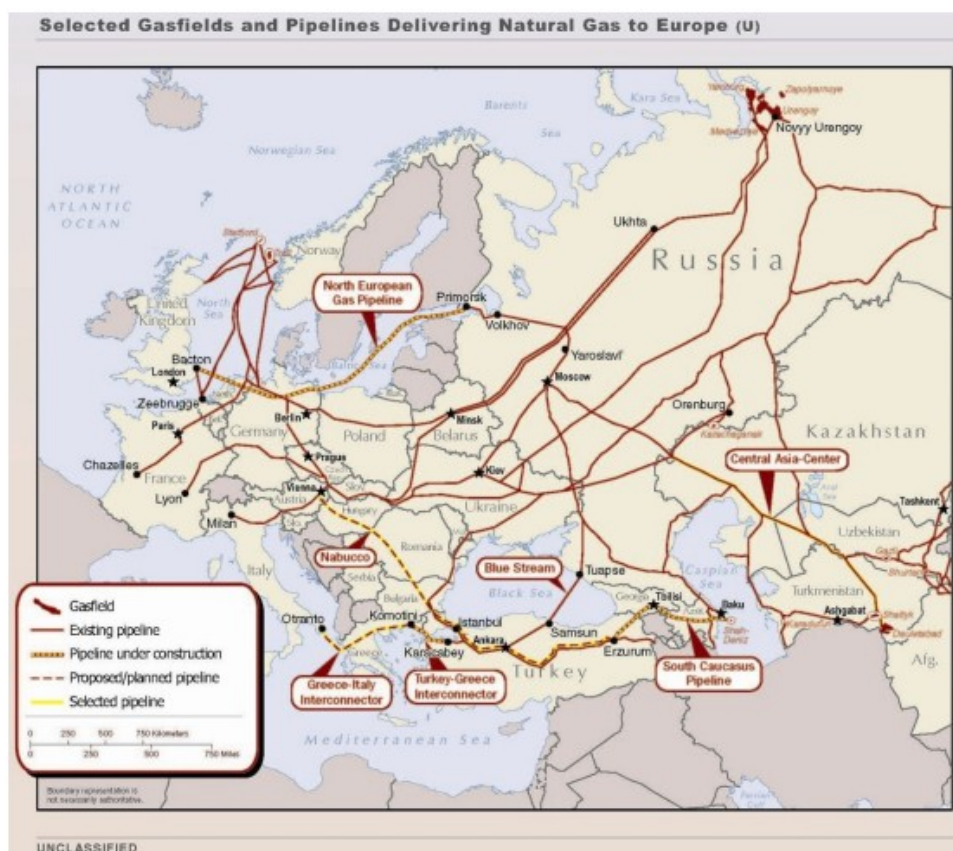
Εικόνα 2. Χάρτης του Ευρωπαϊκού Δικτύου Αγωγών Φυσικού Αερίου (Από την Ιστοσελίδα του ΕΙΑ)
