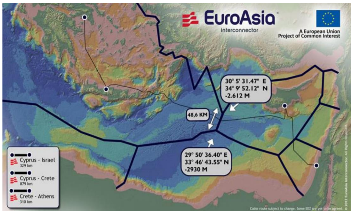
Χάρτης 5: Όδευση Ηλεκτρικής Διασύνδεσης Ισραήλ – Κύπρου – Ελλάδας
